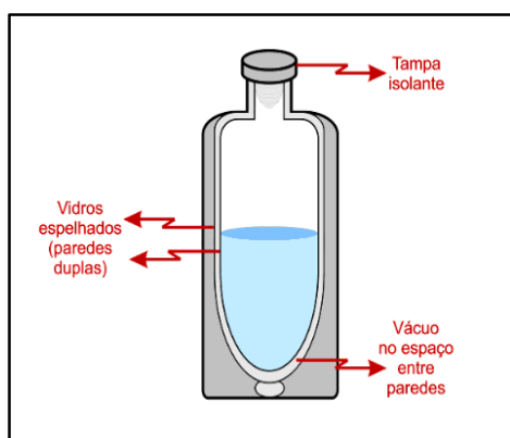
Figura 13 - Esquema de uma garrafa térmica
