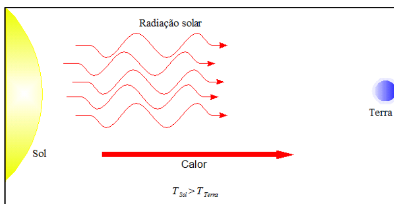
Figura 10 - Transferência de energia térmica pela irradiação solar.
