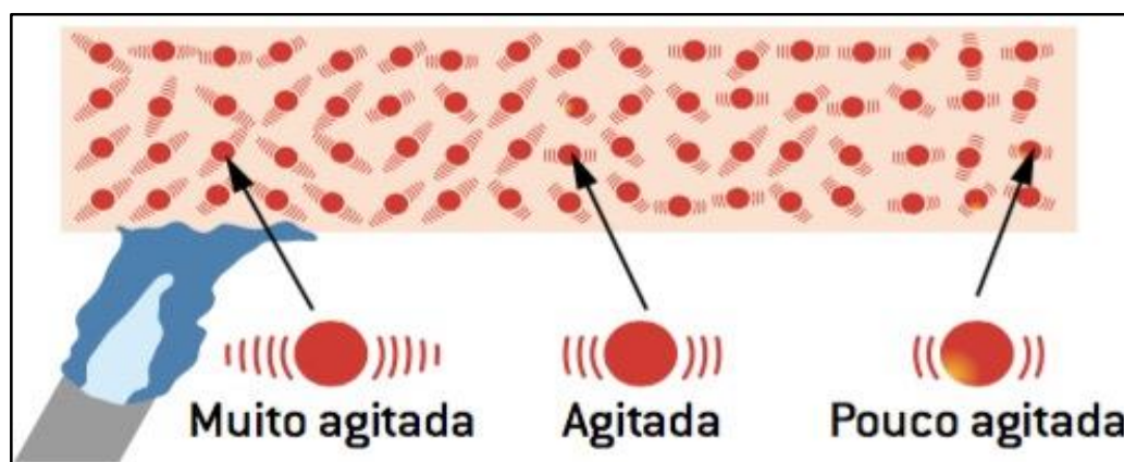
Figura 14 – Representação da propagação de energia térmica entre partículas vizinhas do material.
