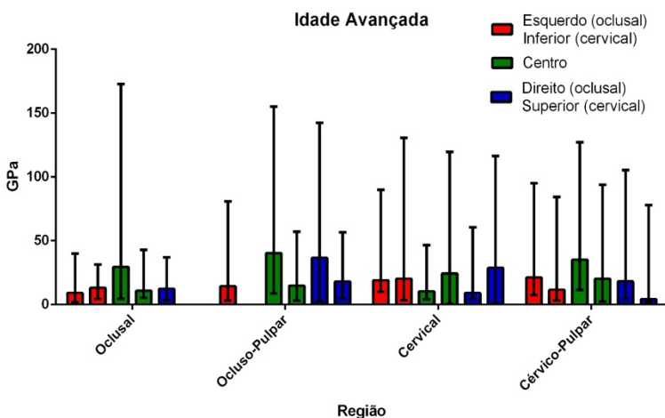
Gráfico 4 - Valores de módulo elástico das regiões mensuradas referentes à dentina de idade avançada.
