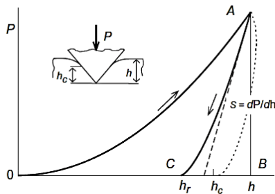
Figura 6 - Gráfico esquemático da obtenção da curva de profundidade de carga em um teste de indentação.
