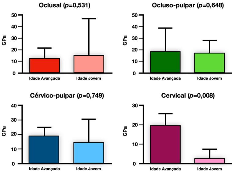
Gráfico 6 - Gráficos comparativos dos módulos elásticos das diferentes regiões das dentinas de idade jovem e avançada. Mann Whitney ( \alpha=0,05 ).
