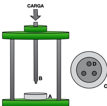
Figura 12 - Dispositivo de ensaio Biaxial (A - Base de posicionamento das amostras; B - Pistão de ponta plana e circular com 1.4mm de diâmetro; C - Base de posicionamento das amostras - vista superior; D - Esferas de apoio - 3.2mm de diâmetro equidistantes 5mm).
