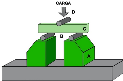
Figura 10 - Dispositivo de ensaio Flexão de 3 pontos; (A - Base; B - Cilindros de apoio com 2mm de diâmetro distantes 11mm; C - Amostra com dimensões 25mm x 2mm x 2mm; D - Cilindro de carga)
