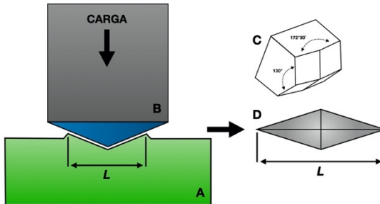
Figura 8 - Esquema microdureza Knoop (HK); (A - Amostra; B - Penetrador Knoop; C - Ponta do penetrador Knoop; D - Geometria do penetrador Knoop; L - Comprimento da penetração).
