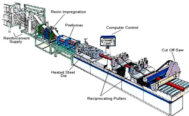
Figura 2 – Esquema do processo de pultrusão.
