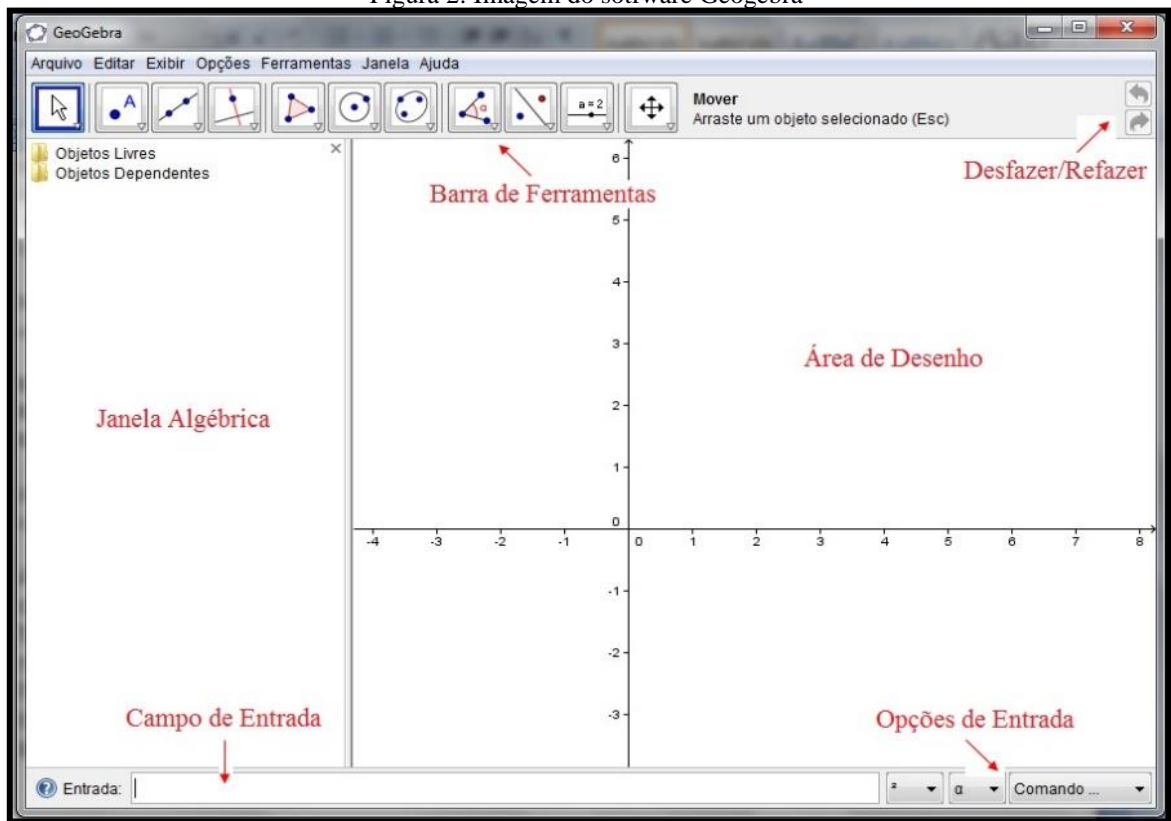
Figura 2: Imagem do software Geogebra
