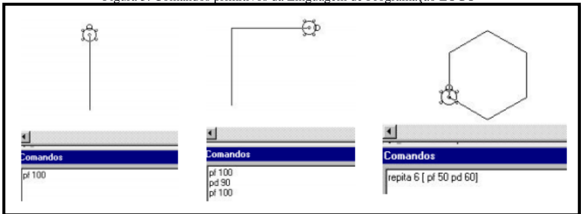
Figura 5: Comandos primitivos da Linguagem de Programação LOGO
