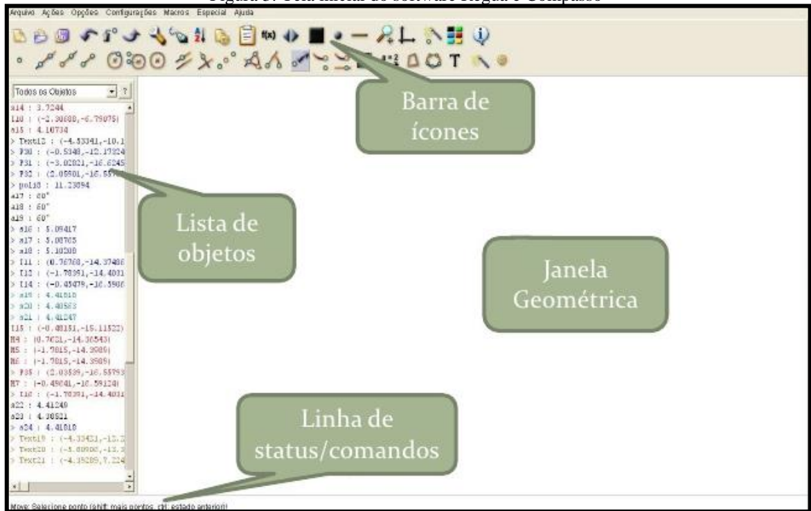
Figura 3: Tela inicial do software Régua e Compasso
