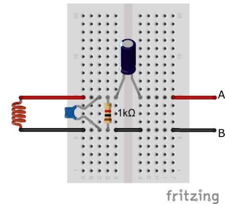
Figura 7: Circuito condicionador de sinal para uso com o cabo de microfone e Audacity.
