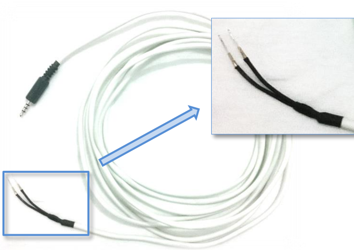
Figura 6: Cabo para ligar o toroide à entrada de microfone do computador.
