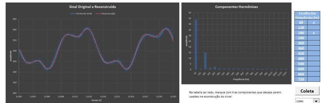
Figura 17: Recorte da tela da planilha Reconstrucao.xlsx. O gráfico à esquerda mostra a curva original e a reconstrução do sinal. O gráfico à direita mostra as componentes harmônicas do sinal. Na tabela, marca-se quais das componentes utilizar para a reconstrução.
