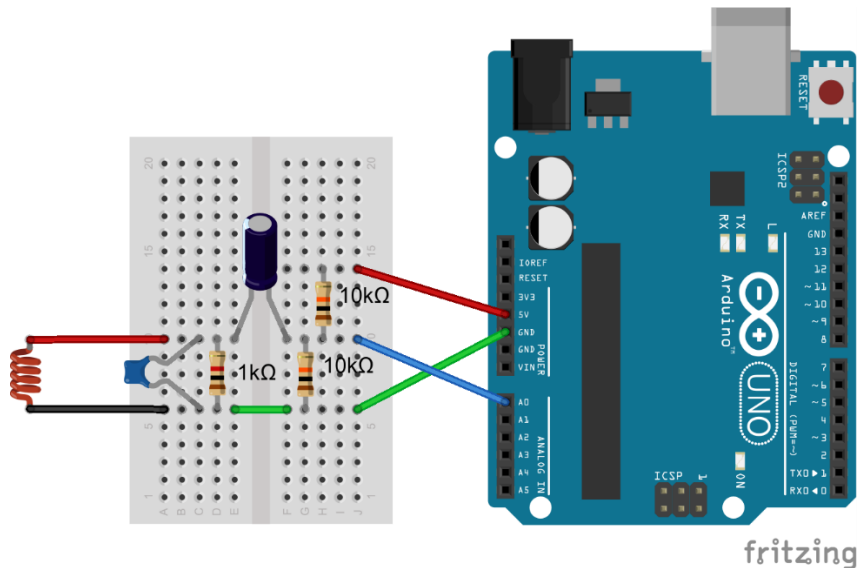
Figura 11: Esquema de montagem do circuito condicionador com o Arduino.
