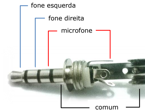
Figura 5: Estrutura do conector P2 de 4 polos.
