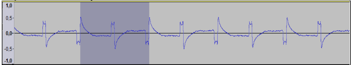
Figura 7 - Forma de onda para um carregador de notebook 64 W / 100-240 V, ligado a uma tomada 220 V. A seleção mostra um ciclo completo.
