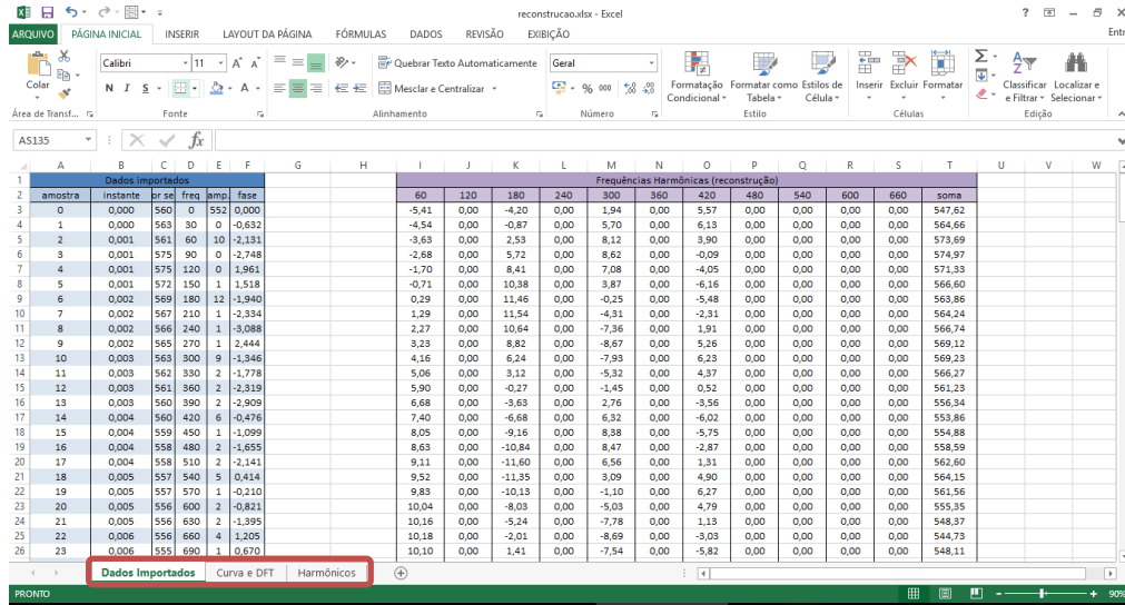
Figura 21 - Tela do arquivo ReconstrucaoSinal.xls para análise do sinal obtido com o programa ColetaCA.py. O arquivo possui três planilhas: Dados Importados, Curva e DFT e Hormônicos.
