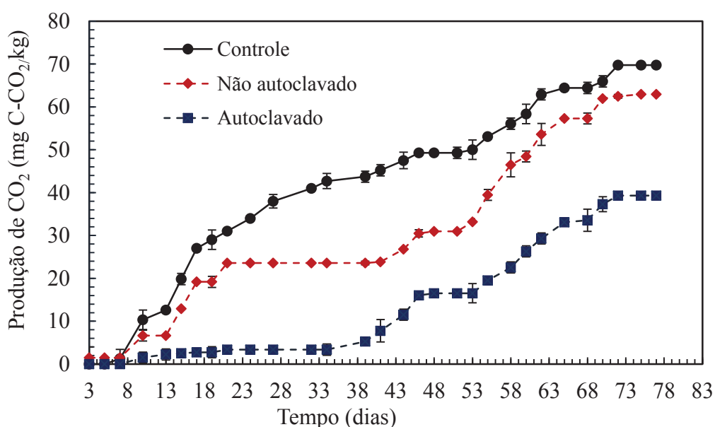
Figura 37 - Acúmulo de CO 2 de diferentes condições experimentais para a nanobiorremediação.
