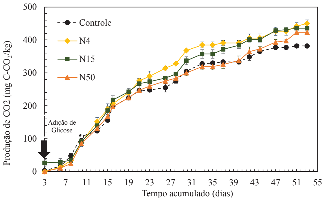
Figura 22 - Acúmulo de CO 2 para diferentes concentrações de nanoferro.
