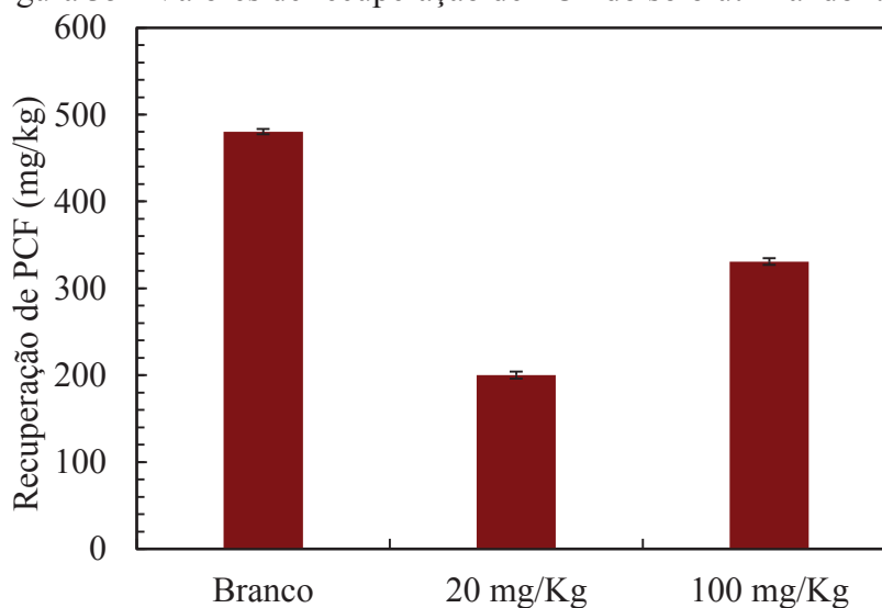
Figura 35 - Valores de recuperação de PCF do solo utilizando \lambda 270 .
