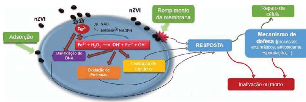
Figura 3 - Mecanismo de Toxicidade do nanoferro.
