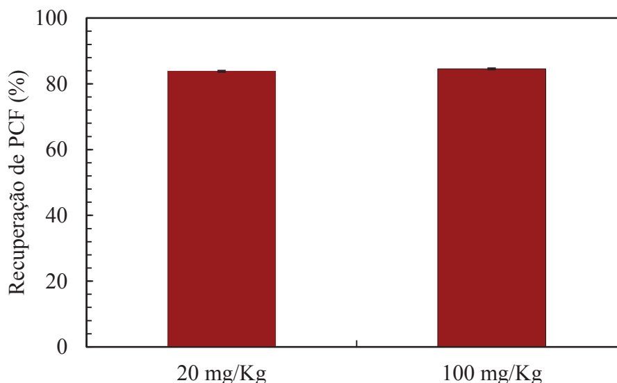
Figura 33 - Valores de recuperação de PCF do solo utilizando \lambda 230 .
